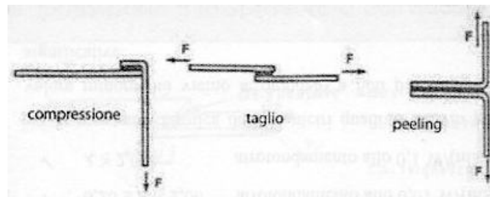
Figura 1 - Principali tipi di incollaggio a sovrapposizione
